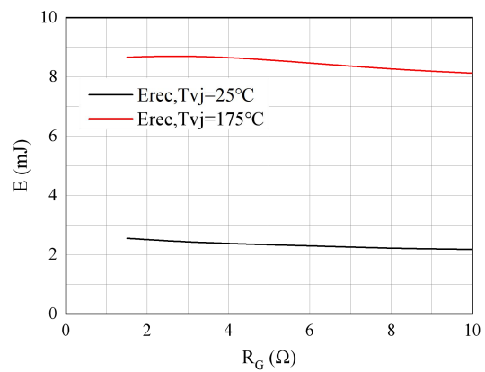
图 12. 开关损耗 二极管 Figure 12. Switching losses of Diode I_F=120A, V_{CE}=600V
